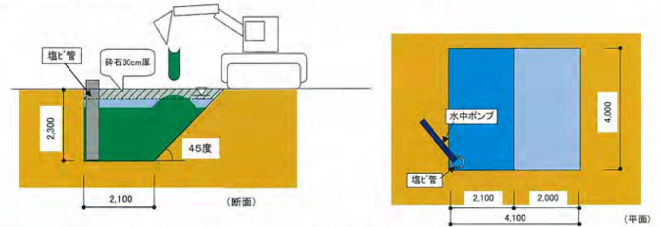
図4 施工試験概略
