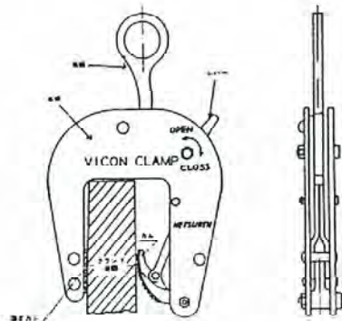
バイコンクランプ
