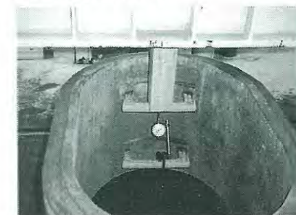
垂直方向荷重試験
