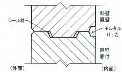
ジョイント部形状
