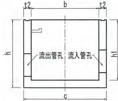
底付 VMB (管取付壁)
