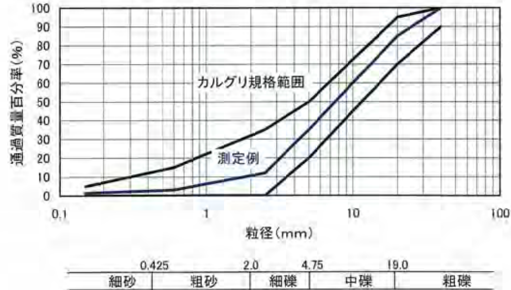
図1 粒度分布
