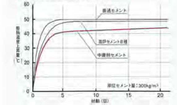
コンクリートの断熱温度上昇の一例
